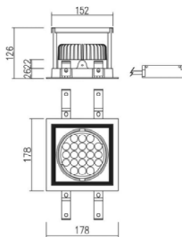
Technische Zeichnung
